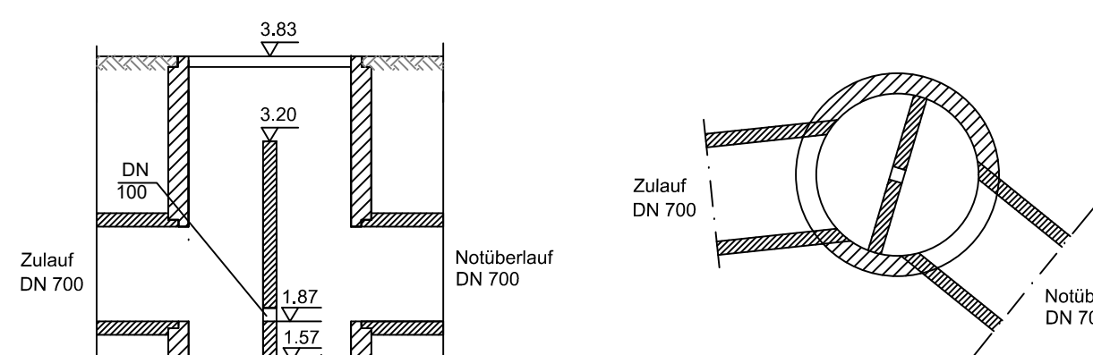
Drosselschacht 01 DN 1200 Schnitt M : 50
