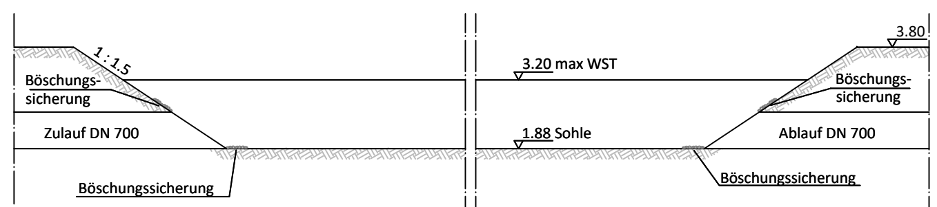
RRB 1 Schnitt 1:100
