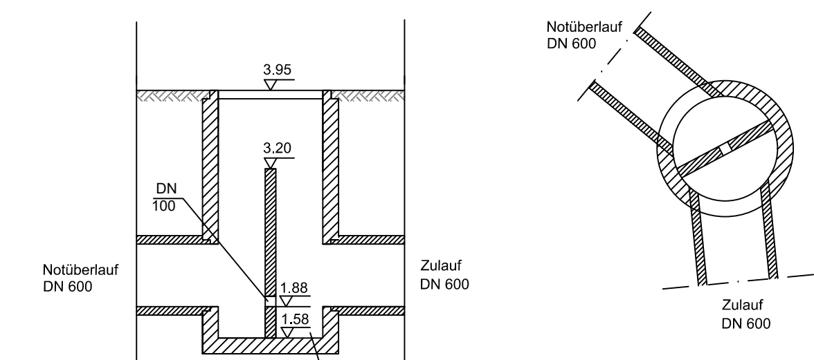
Drosselschacht 02 DN 1000 Schnitt M : 50
