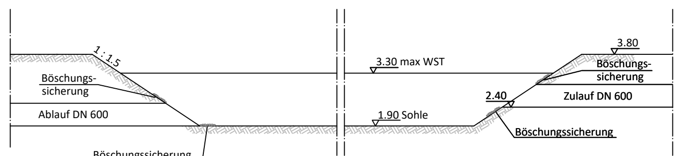
RRB 2 Schnitt 1:100
