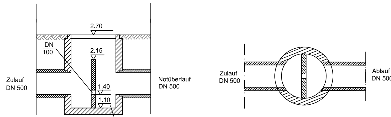
Drosselschacht C DN 1000 Schnitt M : 50
