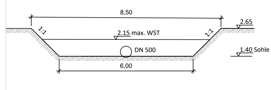
RRG Katjetief Schnitt 1:100
